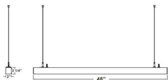
2" (D) x 48" (W) x 2 1/4" (H)
