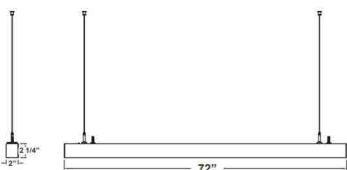
2" (D) x 72" (W) x 2 1/4" (H)
